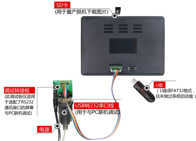
图 1-3 RS232 调试工具图
