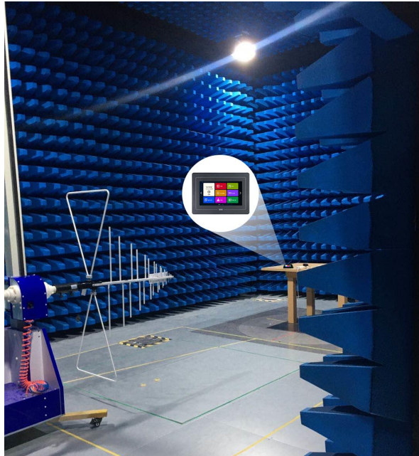
图 5-4 RE 测试图
