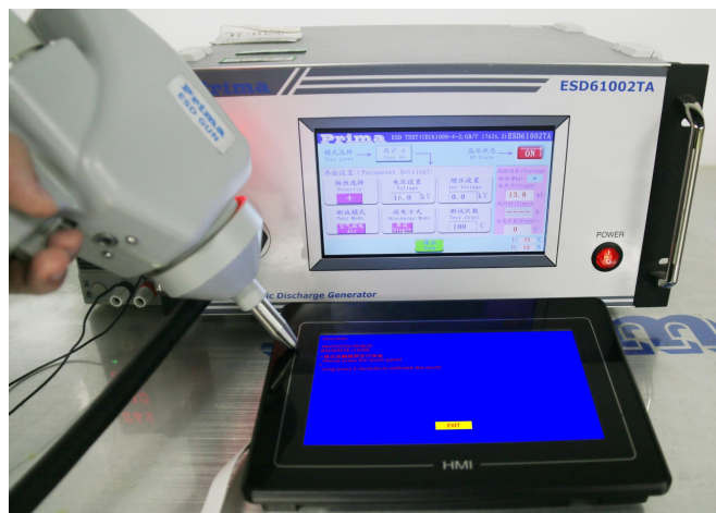
图 5-2 ESD 测试图
